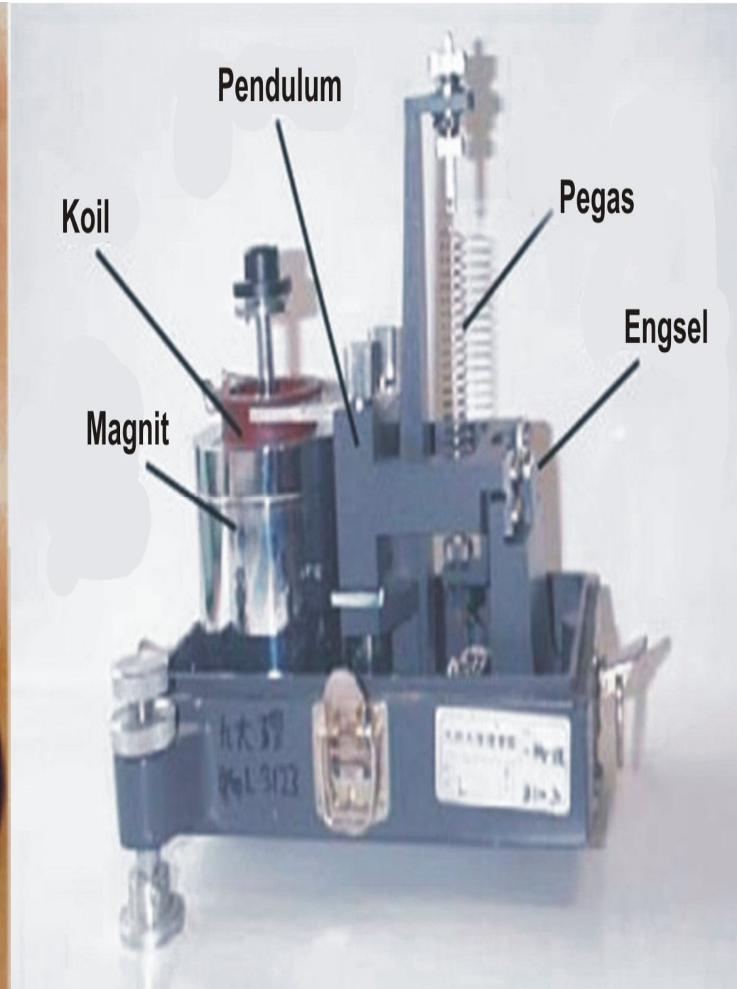
Gambar 16: Seismograf (Alat Pencatan Gempa Bumi)
